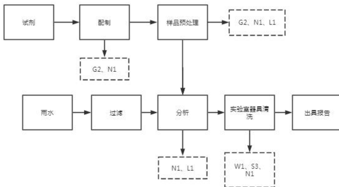
图 5-2 雨水径流的净化效果研究工艺流程
