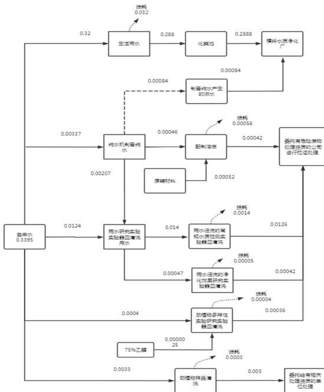
图 5-5 项目水平衡图 (单位: \text{m}^3/\text{d} )
