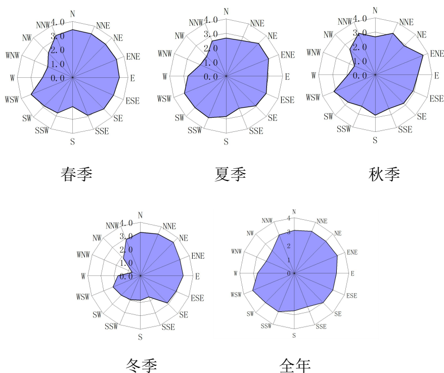
图 2-1 各季度及全年风速图
