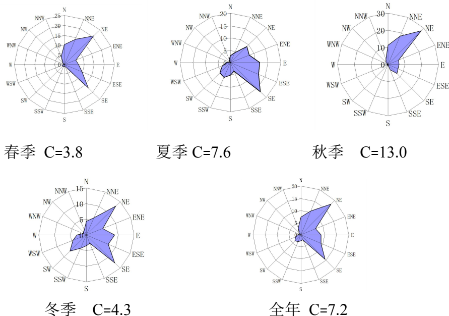
图 2-2 各季度及全年风向玫瑰图
